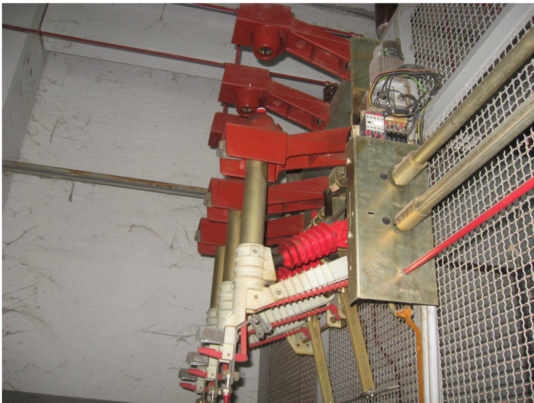
Figura 2 IMPIANTO DI TANCA MOLINO sostituzione sezionatori
